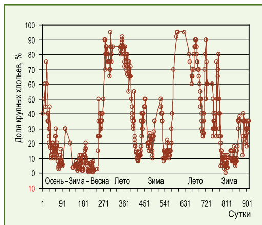
Рис. 2. Сезонная изменчивость фракционного состава ила
